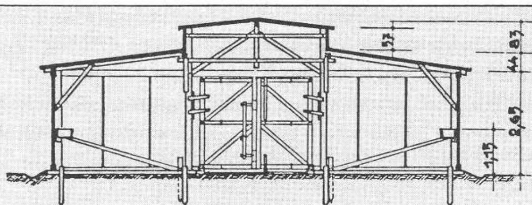
QUERSCHNITT
